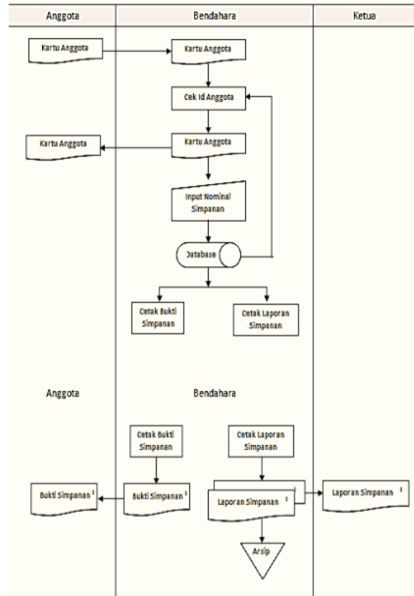
Gambar 5 Flowmap Simpanan yang diusulkan
