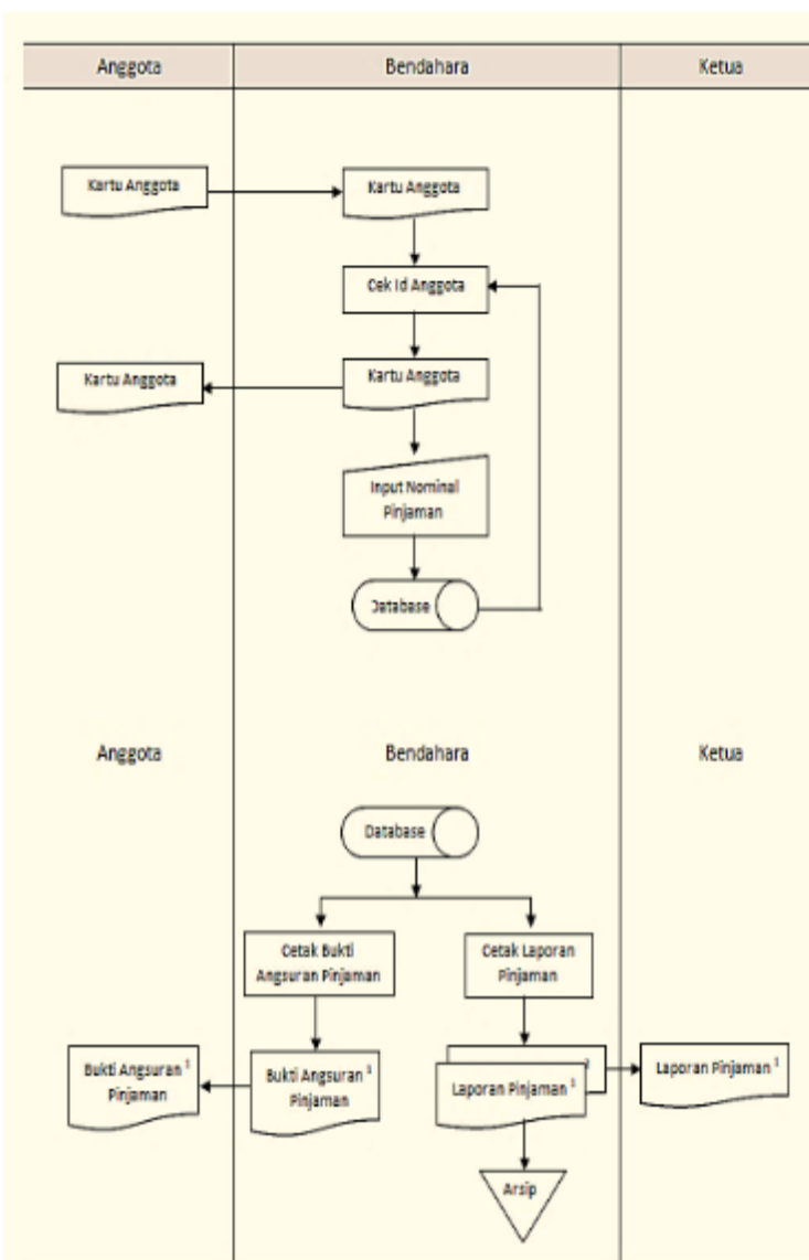
Gambar 6 Flowmap Pinjaman yang diusulkan
