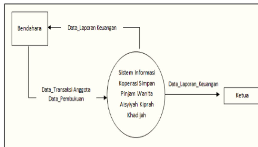
Gambar 8 Diagram Konteks
